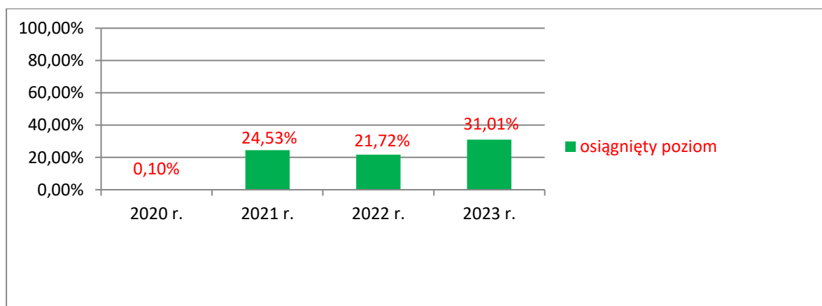
Rys. 3. Osiągnięty poziom składowania odpadów komunalnych z terenu miasta.
