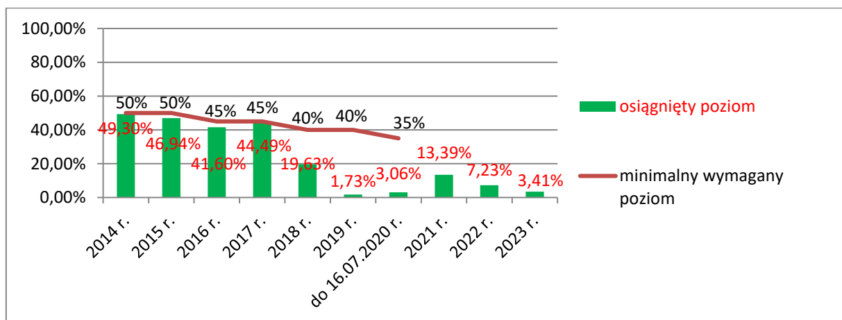
Rys. 2. Osiągnięty poziom ograniczenia masy odpadów komunalnych ulegających biodegradacji przekazywanych do składowania z terenu miasta.
